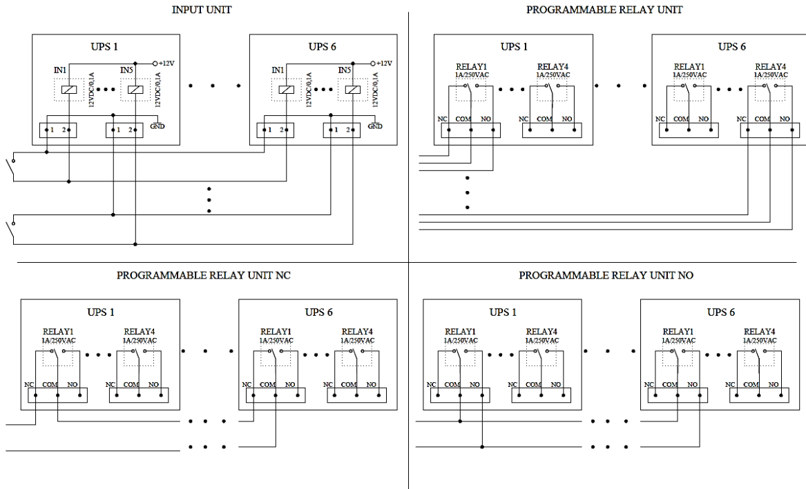
Rysunek 2. Sposób łączenia obwodów sterujących i sygnalizacyjnych w zasilaczach POWERLINE GREEN 33 10-60 kVA.
