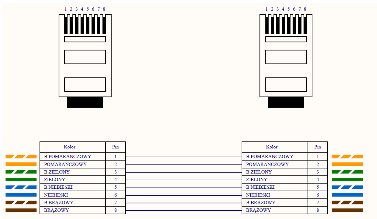
Rysunek 3. Sposób zakończenia przewodów komunikacyjnych w zasilaczach POWERLINE GREEN 33 10-60 kVA w układzie równoległym / redundanтным.
