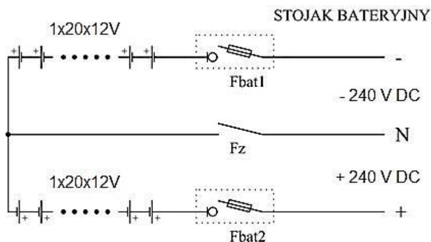
Rysunek 3. Schemat podłączenia stojaka bateryjnego do zasilacza POWERLINE DARK 33 60-200 kVA
