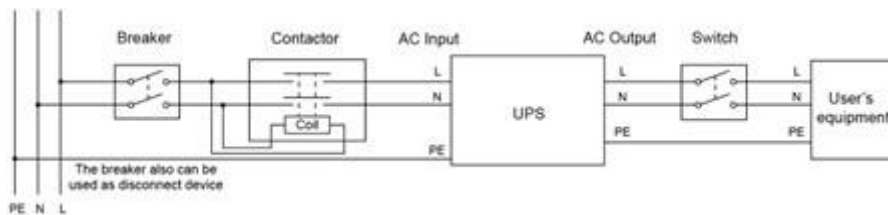
Rysunek 7: Podłączenie zasilacza w konfiguracji 1/1
