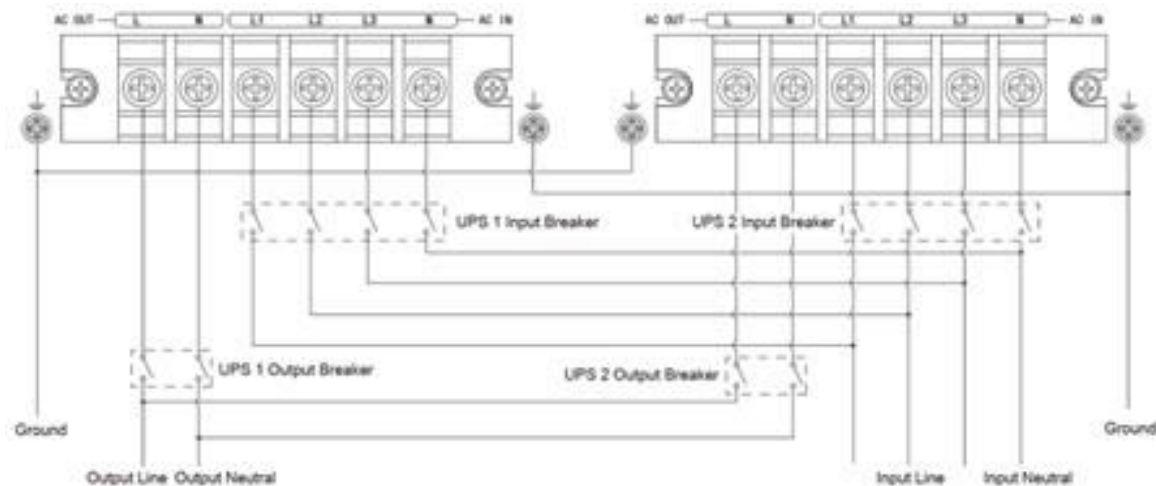
Rysunek 16: Schemat instalacji elektrycznej układu równoległego zasilaczy POWERLINE MULTI 10-11/31
