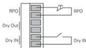
Rysunek 17: Styki bezpotencjałowe
