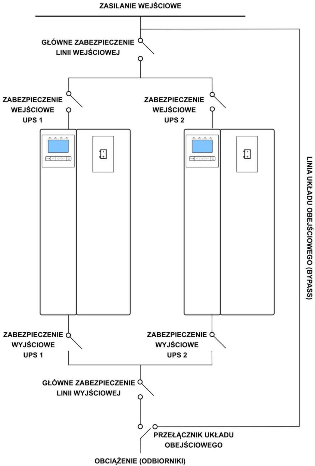
Rysunek 15: Schemat połączenia układu równoległego zasilaczy POWERLINE MULTI 10-11/31
