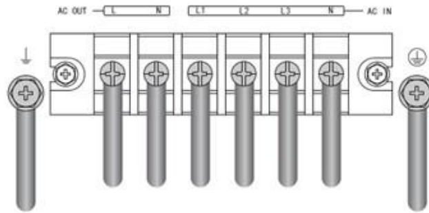
Rysunek 4: Elementy przyłączeniowe zasilacza
