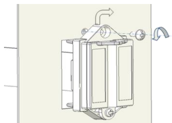
Rysunek 10: Demontaż maskownicy
