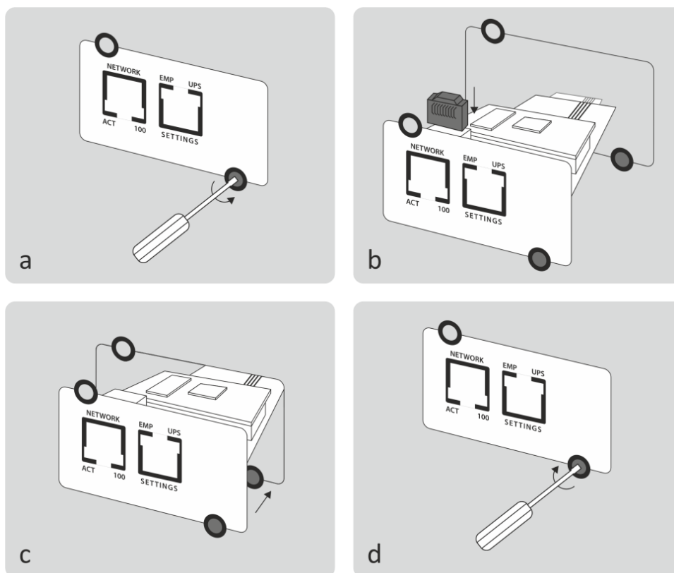
Rysunek 18: Montaż karty zarządzającej
