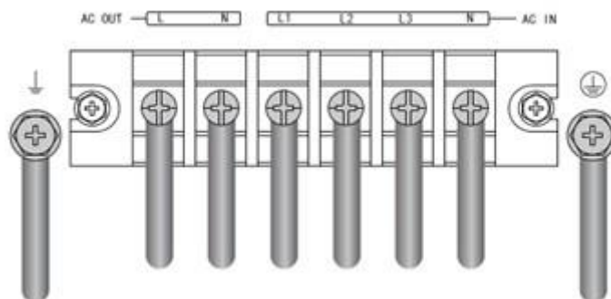
Rysunek 5: Podłączenie zasilacza w konfiguracji 3/1
