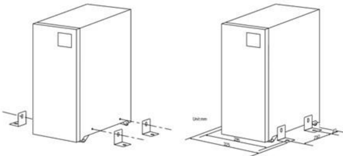
Rysunek 3: Montaż uchwytów
