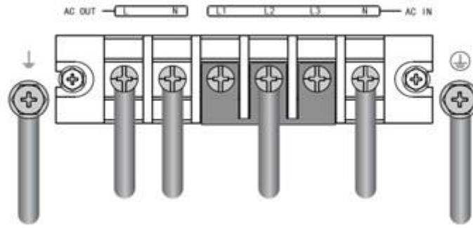
Rysunek 6: Podłączenie zasilacza w konfiguracji 1/1
