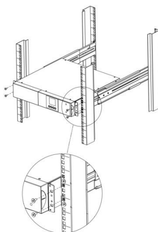
Rysunek 22: Montaż zasilacza w szafie
