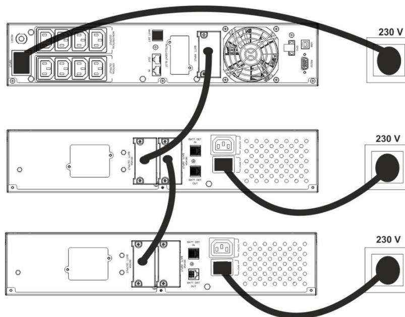
Rysunek 24: Połączenie zasilacza w raz z modułami
