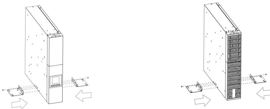
Rysunek 14: Montaż stopek do zasilacza i modułu baterijnego
