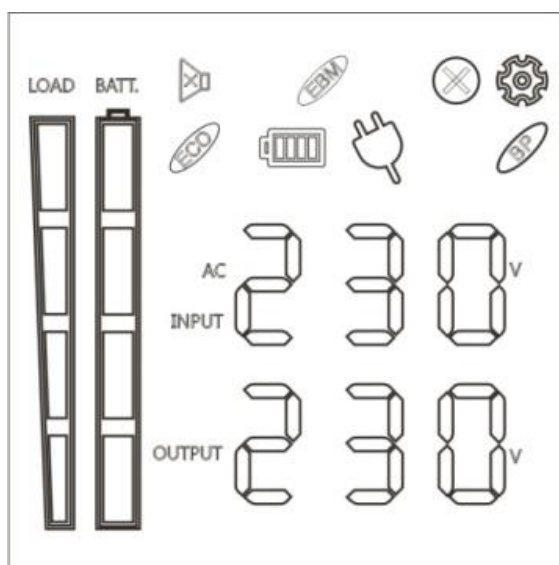
Rysunek 7: Widok wyświetlacza LCD z ikonami informacyjnymi (wersja RACK)
