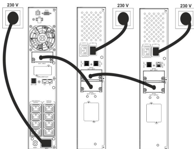
Rysunek 18: Połączenie zasilacza wraz z modułami
