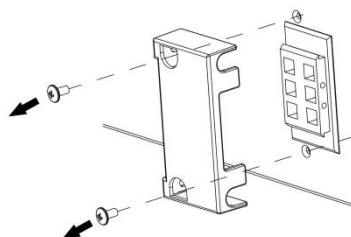
Rysunek 16: Demontaż osłony gniazda
