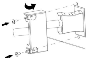
Rysunek 17: Montaż osłony gniazda
