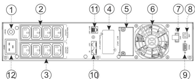
Rysunek 2: Widok panelu tylnego POWERLINE RT PLUS 2000
