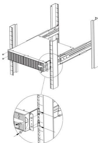
Rysunek 23: Montaż modułu bateryjnego w szafie
