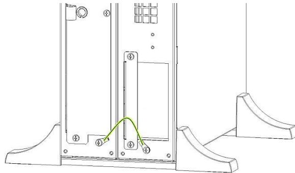
Rysunek 22: Połączenie przewodu PE
