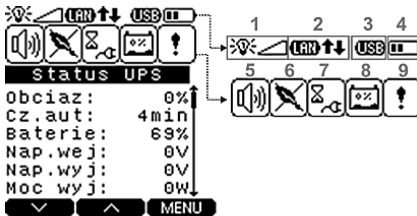
Rysunek 6: Widok wyświetlacza LCD z ikonami informacyjnymi
