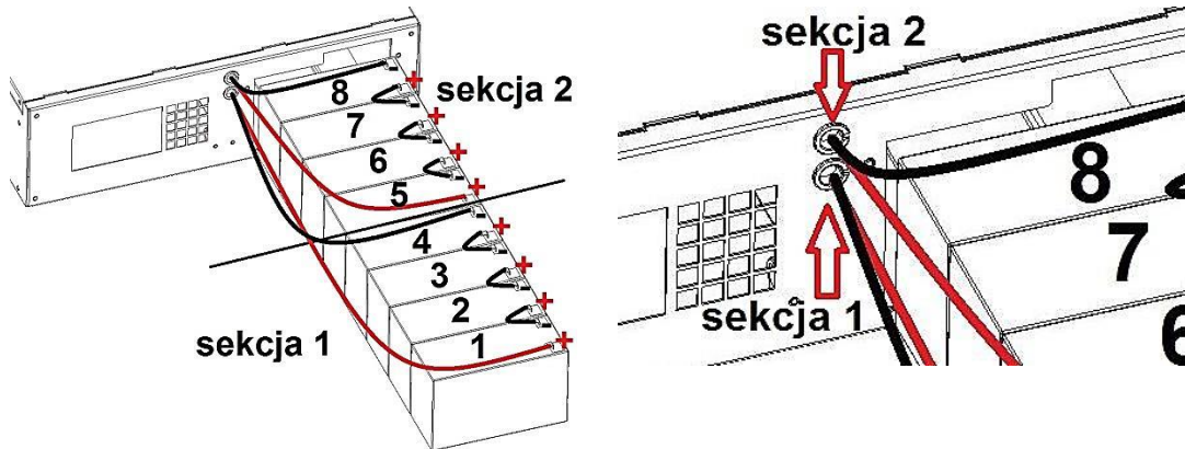
Rysunek 44: Układ i połączenie akumulatorów
