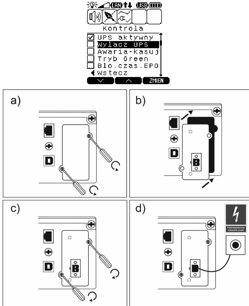
Rysunek 49: Montaż karty w zasilaczu
