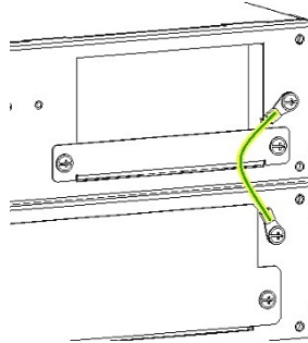
Rysunek 34: Połączenie przewodu PE
